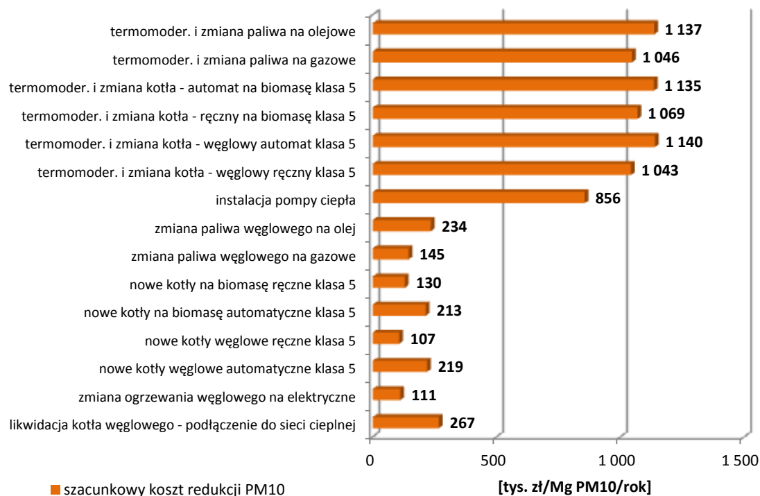
Rysunek 72. Porównanie szacunkowych, średnich wskaźników kosztów redukcji pyłu zawieszony PM10 z indywidualnych systemów grzewczych
