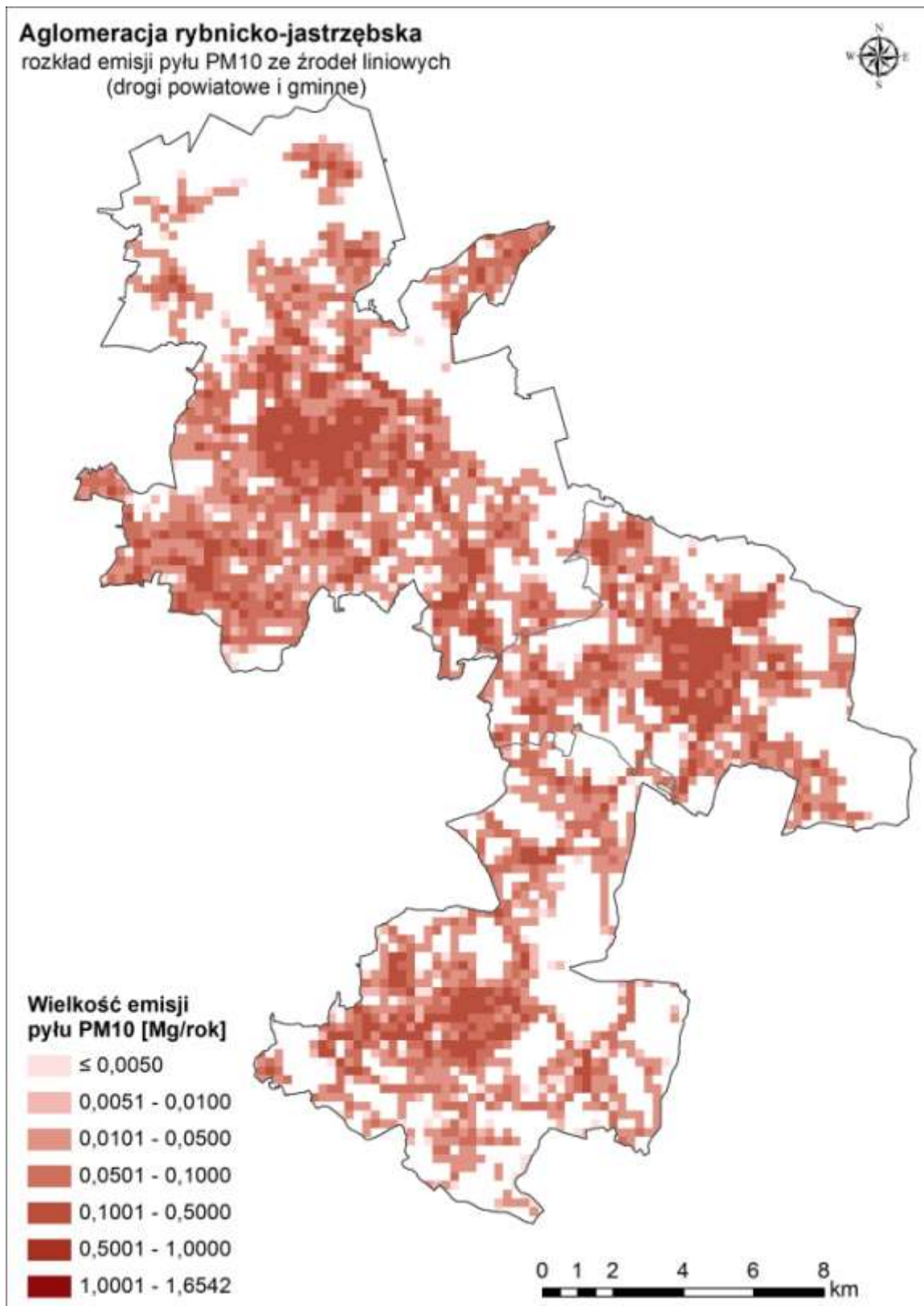
Rysunek 154. Lokalizacja i wielkość emisji pyłu PM 10 z dróg powiatowych i gminnych w aglomeracji rybnicko-jastrzębskiej w roku bazowym 2015
