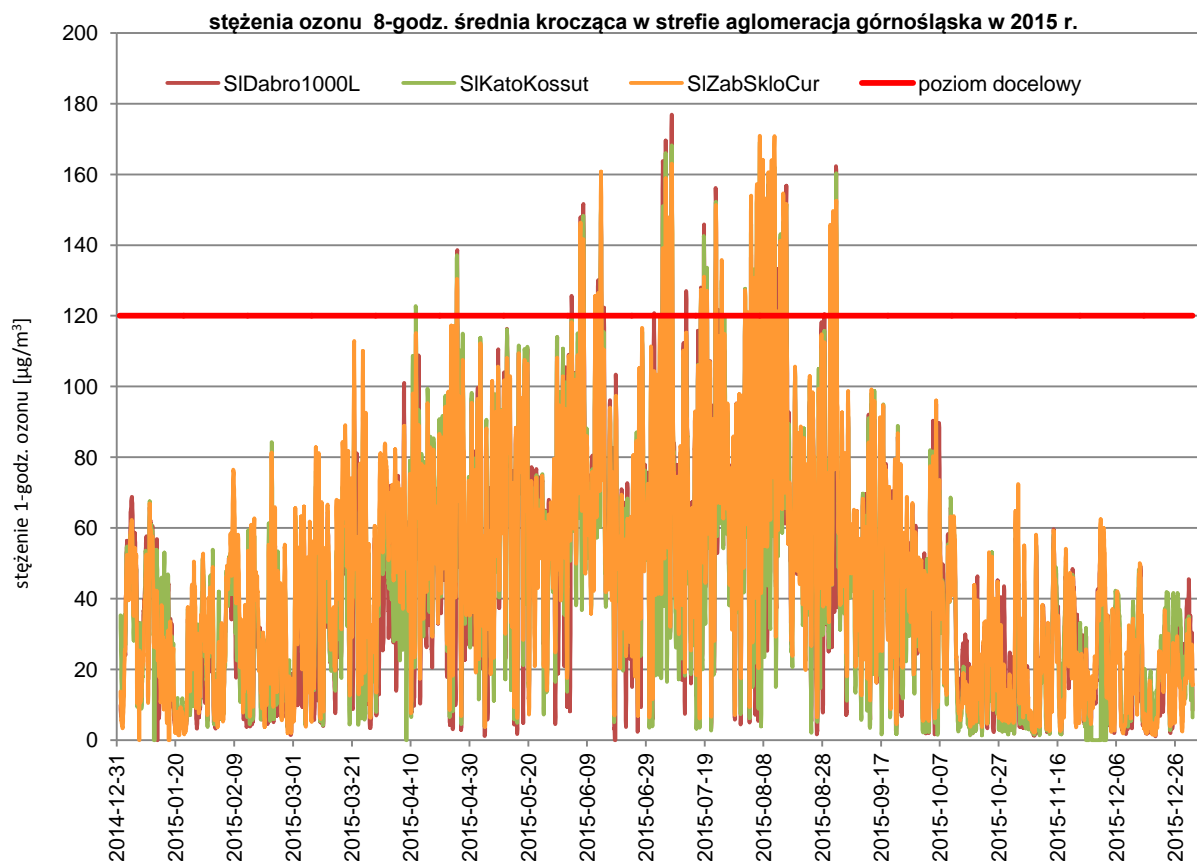
Rysunek 16. Przebieg zmienności 8-godzinnej średniej kroczącej dla ozonu w strefie aglomeracja górnośląska w 2015 roku 78
