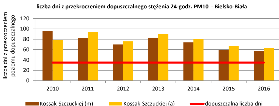
Rysunek 29. Liczba dni z przekroczeniem poziomu dopuszczalnego 24 godzinnego pyłu PM10 w latach 2010-2016 w punktach pomiarowych w strefie miasto Bielsko-Biała 104
