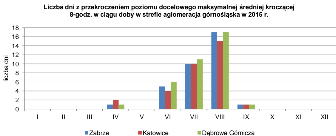
Rysunek 15. Liczba dni z przekroczeniem poziomu docelowego maksymalnej średniej kroczącej 8-godz. dla ozonu w ciągu doby powyżej wartości 120 \mu\text{g}/\text{m}^3 w roku 2015 w punktach pomiarowych na terenie aglomeracji górnośląskiej 77
