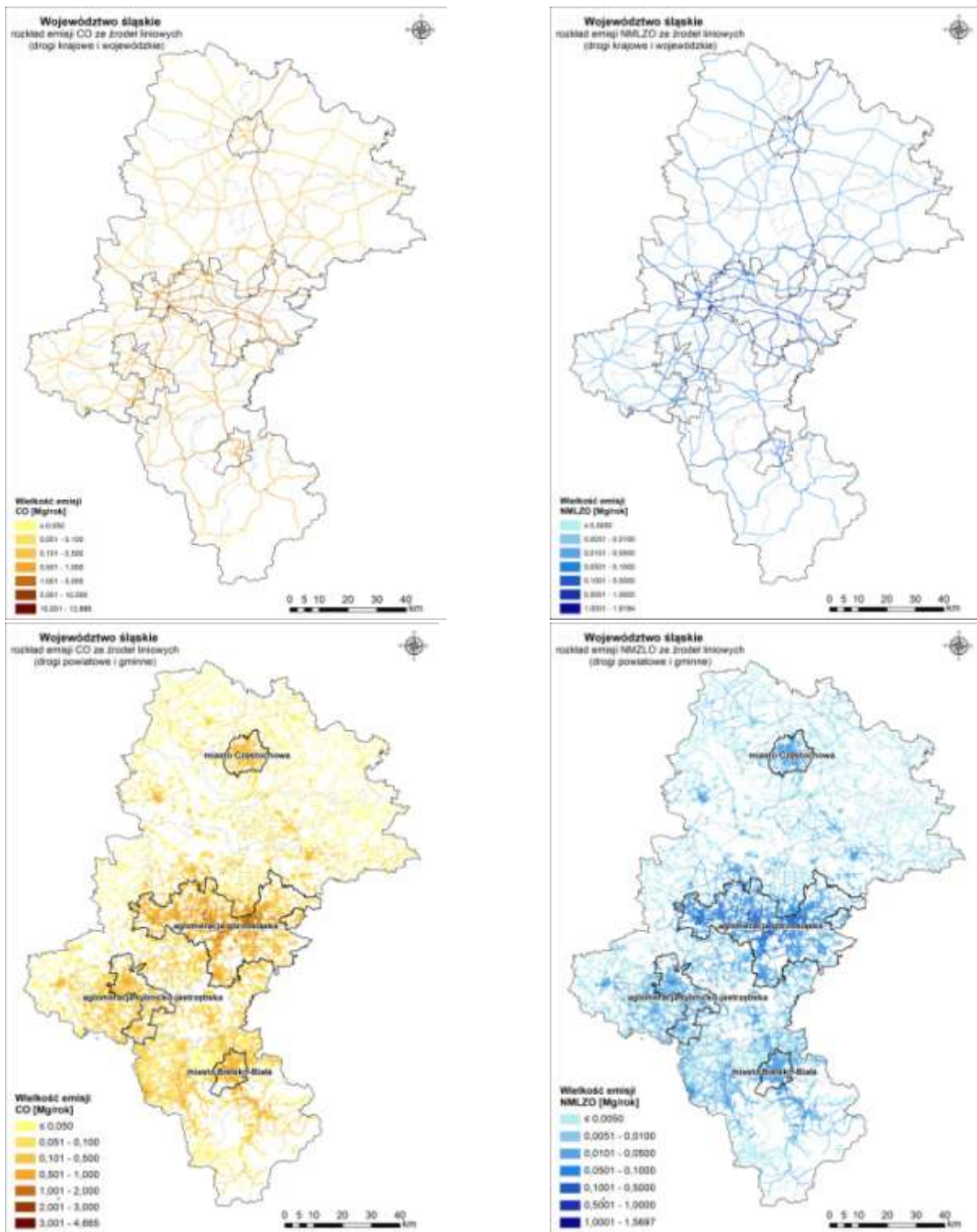
Rysunek 93. Rozkład przestrzenny emisji prekursorów pyłu i ozonu ze źródeł liniowych w siatce obliczeniowej w województwie śląskim w roku bazowym 2015
