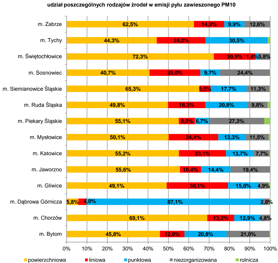
Rysunek 100. Udział poszczególnych rodzajów źródeł w emisji pyłu zawieszanego PM10 z terenu powiatów strefy aglomeracja górnośląska w roku bazowym 2015
