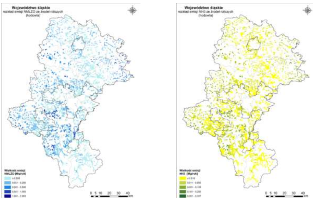
Rysunek 96. Rozkład przestrzenny emisji prekursorów pyłu i ozonu z hodowli w siatce obliczeniowej na terenie województwa śląskiego w roku bazowym 2015
