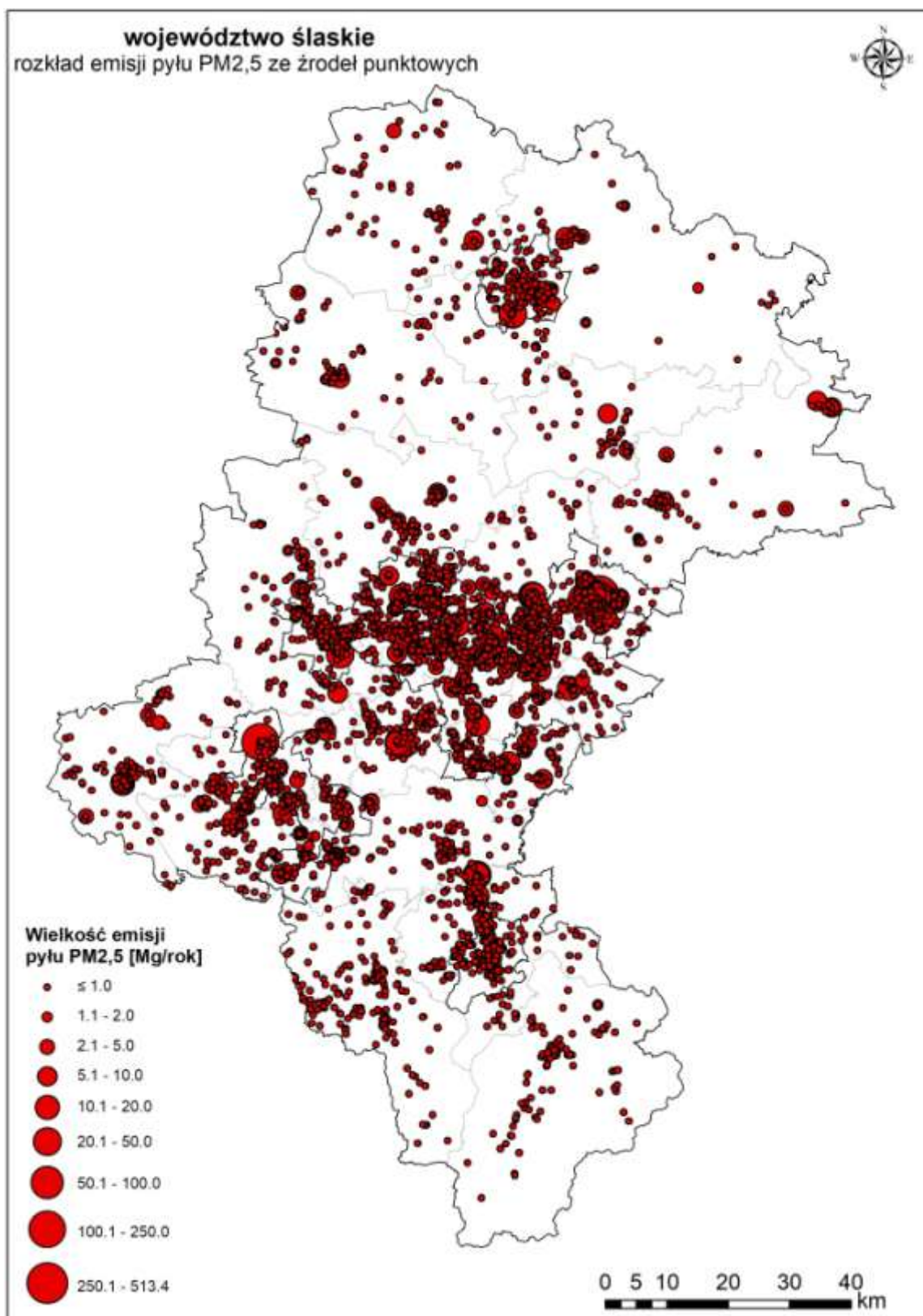
Rysunek 130. Lokalizacja i wielkość emisji pyłu zawieszony PM 2,5 ze źródeł punktowych w województwie śląskim w roku bazowym 2015
