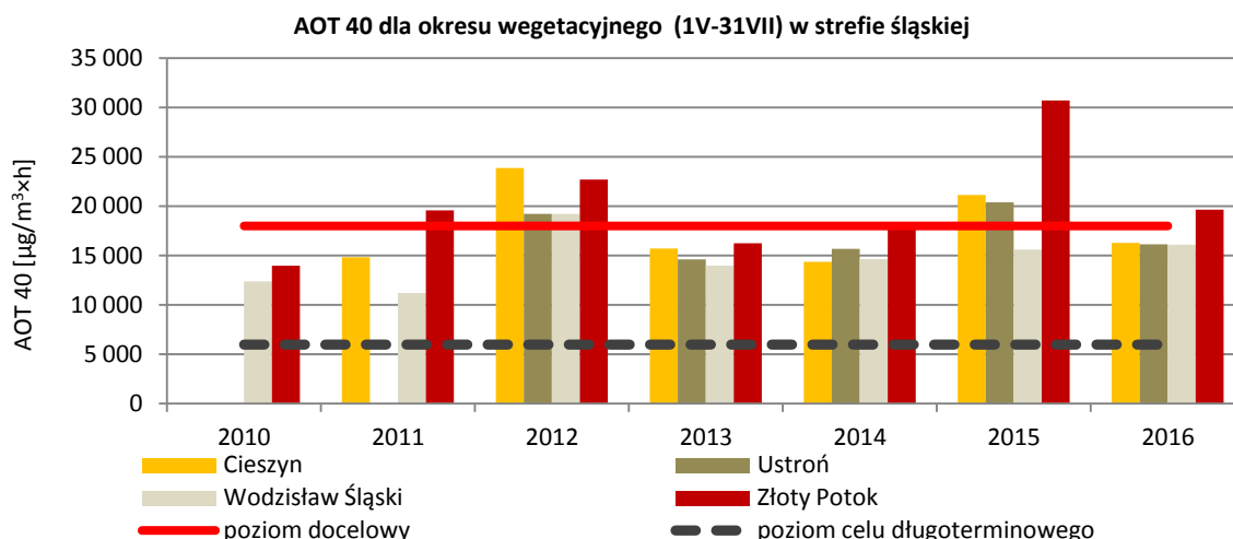
Rysunek 50. Wskaźnik AOT 40 dla poziomu docelowego i celu długoterminowego obliczony dla okresu wegetacyjnego (1V-31VII) w punktach pomiarowych w strefie śląskiej dla lat 2010-2016 146
