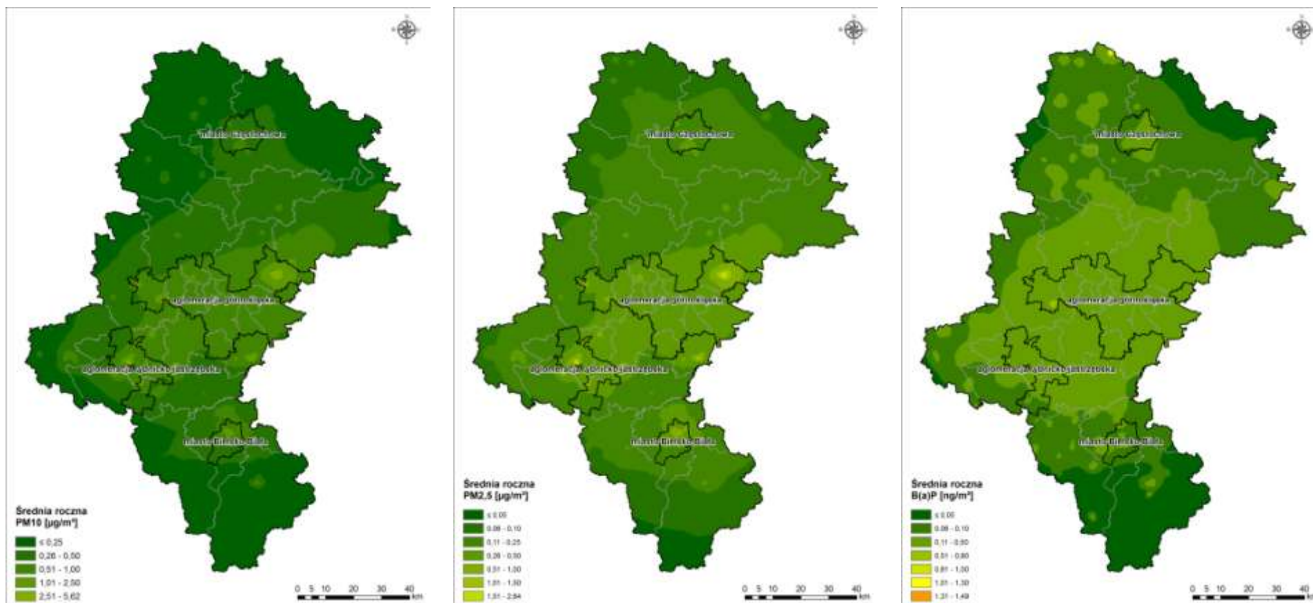
Rysunek 64. Rozkład stężeń średniorocznych pyłu PM10, PM2,5 oraz B(a)P generowanych przez źródła punktowe w województwie śląskim 154
