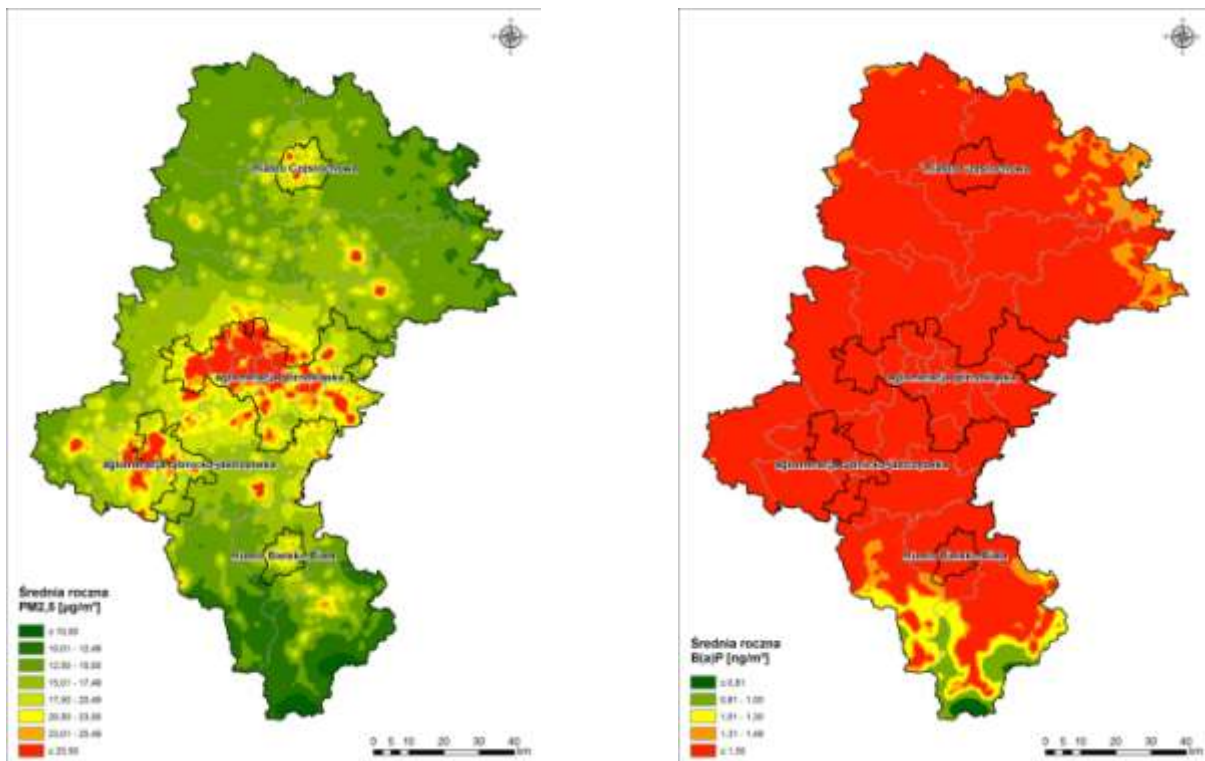
Rysunek 54. Rozkład przestrzenny stężeń średniorocznych pyłu zawieszonego PM 2,5 i benzo(a)pirenu na terenie województwa śląskiego w roku bazowym 2015
