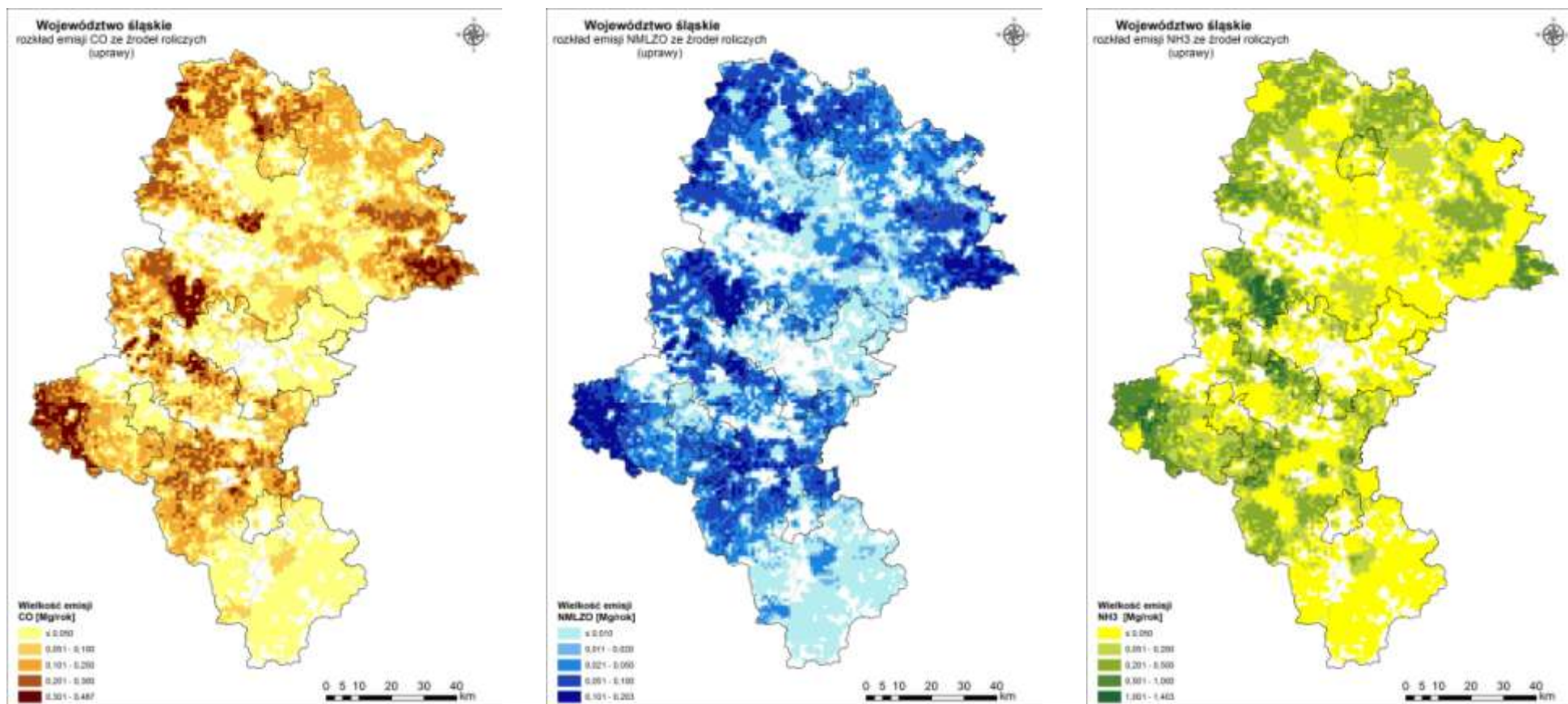
Rysunek 98. Rozkład przestrzenny emisji prekursorów pyłu i ozonu z obszarów upraw w siatce obliczeniowej na terenie województwa śląskiego w roku bazowym 2015
