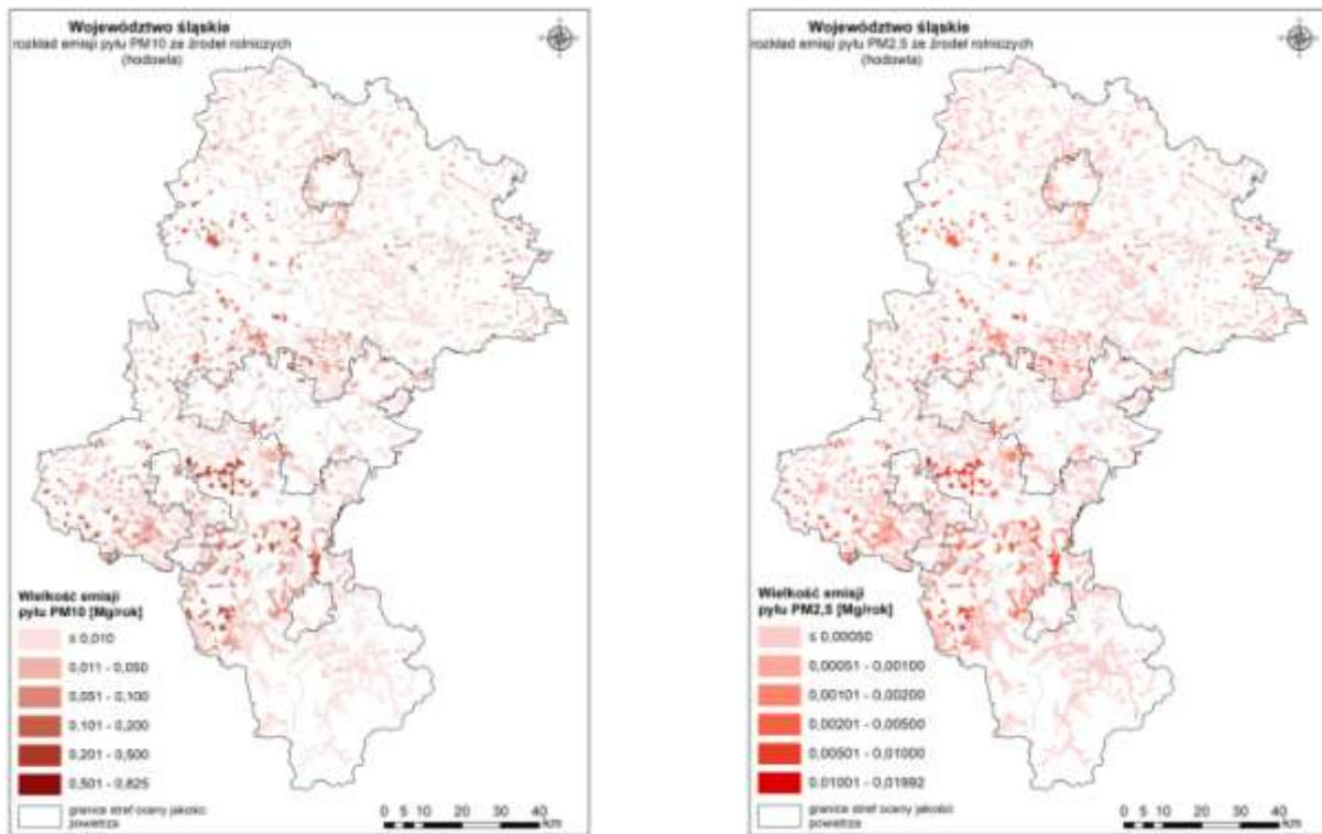
Rysunek 95. Rozkład przestrzenny emisji pyłu zawieszzonego PM10 i PM2,5 z hodowli w siatce obliczeniowej na terenie województwa śląskiego w roku bazowym 2015
