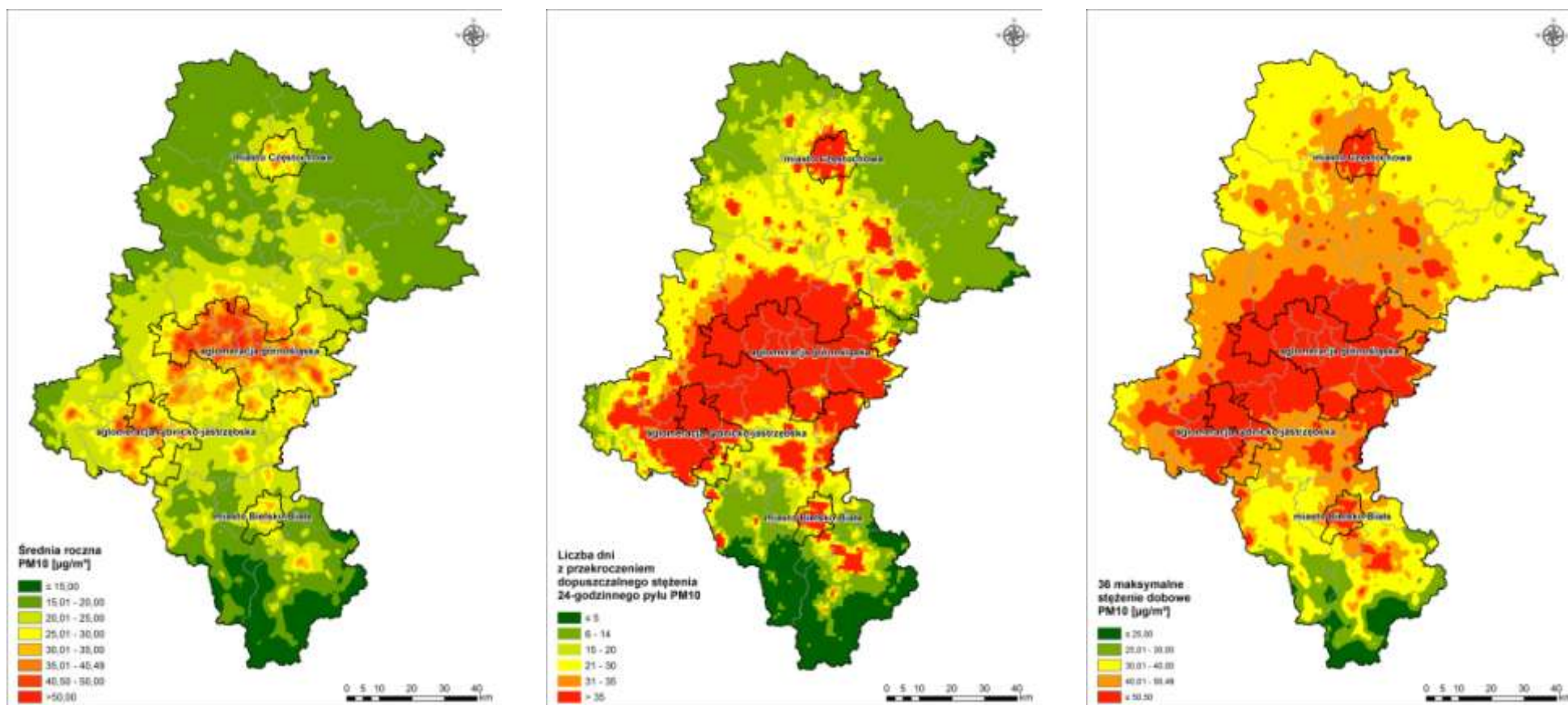
Rysunek 53. Rozkład przestrzenny wielkości stężeń średniorocznych, liczby dni z przekroczeniem dopuszczalnego stężenia dobowego oraz 36-te maksymalne stężenie dobowe dla pyłu zawieszony PM10 na terenie województwa śląskiego w roku bazowym 2015
