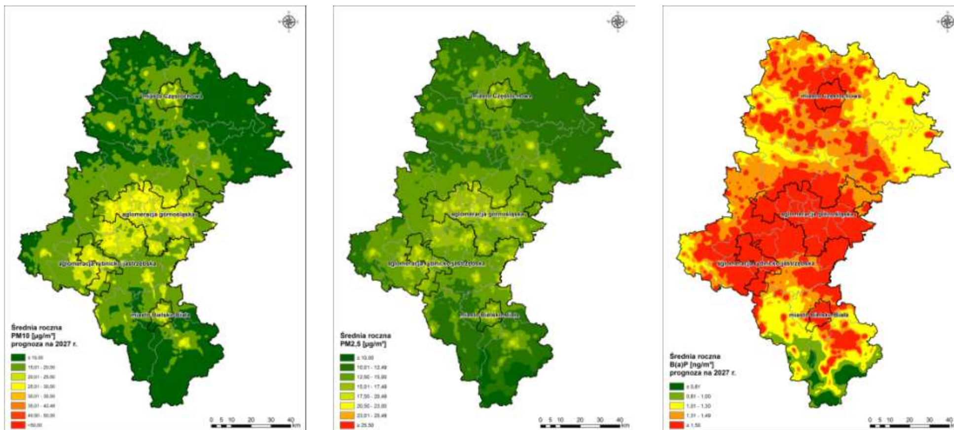
Rysunek 120. Rozkład przestrzenny stężeń średniorocznych pyłu zawieszonego PM10 i PM2,5 oraz benzo(a)pirenu w województwie śląskim w roku prognozy 2027
