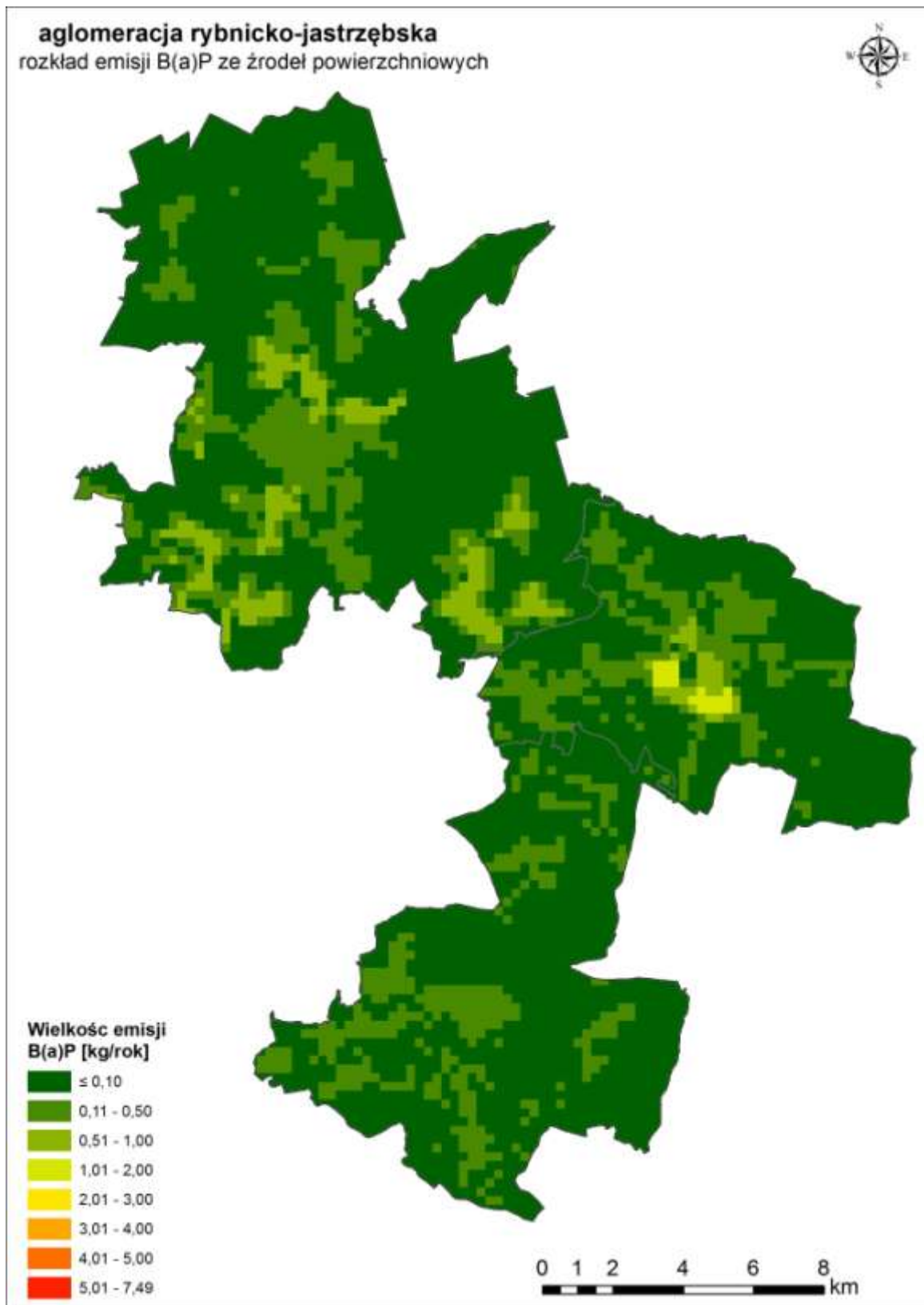
Rysunek 139. Lokalizacja i wielkość emisji B(a)P ze źródeł powierzchniowych w aglomeracji rybnicko-jastrzębskiej w roku bazowym 2015 272
