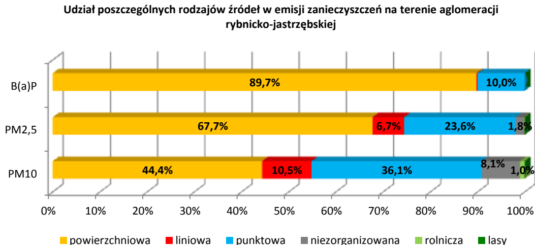
Rysunek 105. Procentowy udział poszczególnych rodzajów źródeł w sumarycznej emisji pyłu PM10, PM2,5 i B(a)P dla strefy aglomeracja rybnicko-jastrzębska w roku bazowym 2015 208
