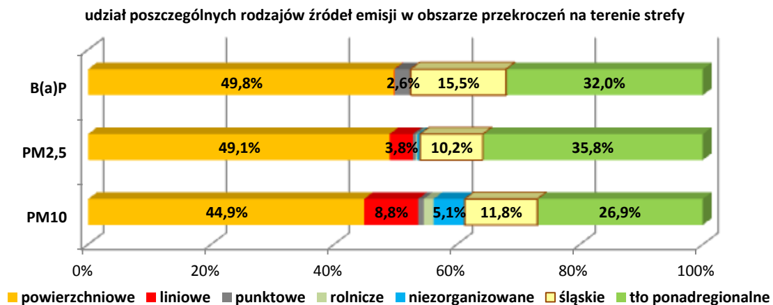
Rysunek 61. Udziały poszczególnych rodzajów źródeł emisji w wielkości stężeń analizowanych zanieczyszczeń w obszarze przekroczeń na terenie strefy śląskiej 151
