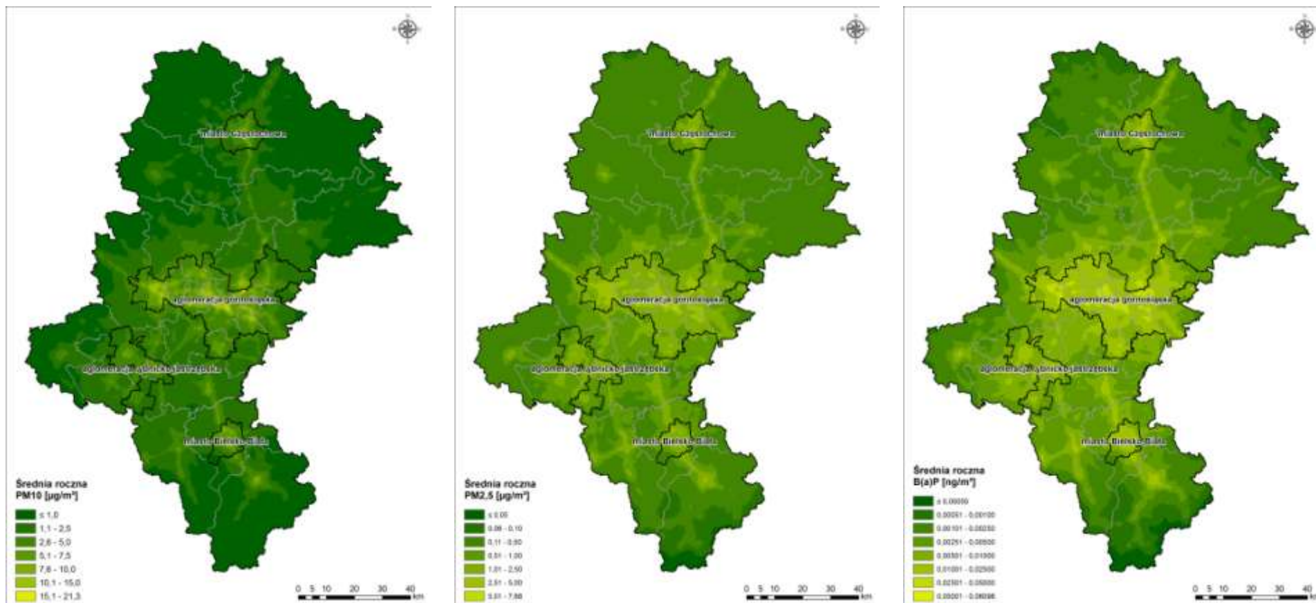
Rysunek 63. Rozkład stężeń średniorocznych pyłu PM10, PM2,5 oraz B(a)P generowanych przez źródła liniowe w województwie śląskim 153
