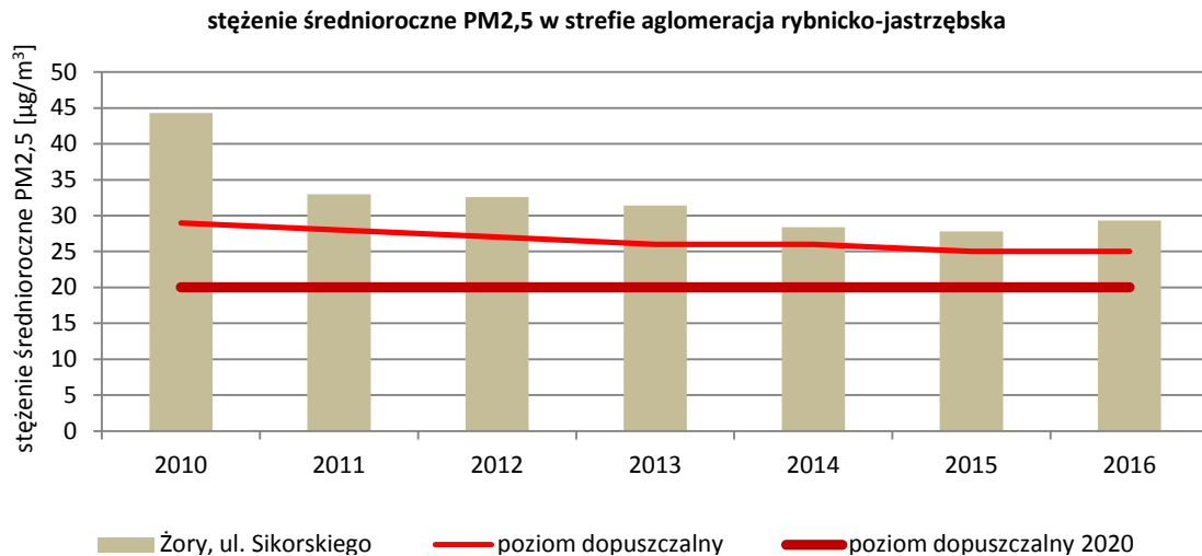
Rysunek 21. Wyniki pomiarów stężeń średniorocznych pyłu PM 2,5 w latach 2010-2016 w strefie aglomeracji rybnicko-jastrzębska 89
