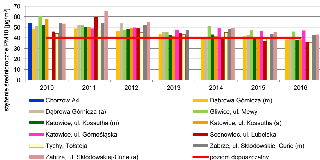
stężenie średnioroczne pyłu zawieszonego PM10 w strefie aglomeracja górnośląska
