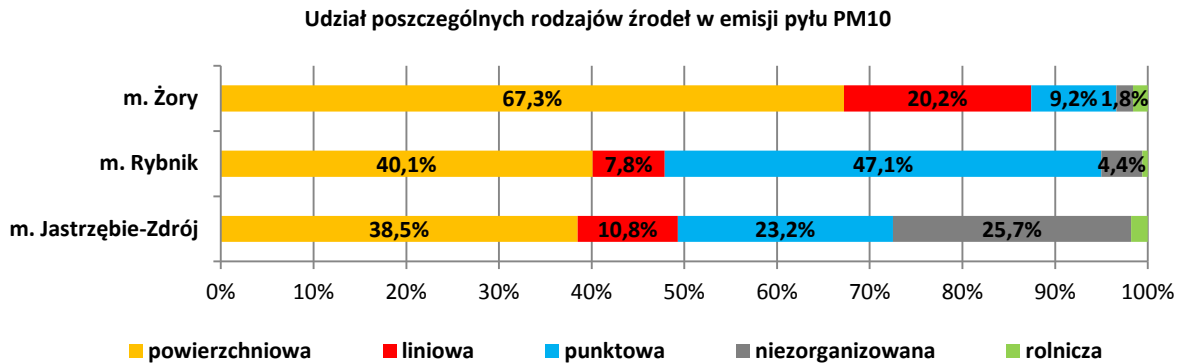
Rysunek 106. Procentowy udział poszczególnych rodzajów źródeł w sumarycznej emisji pyłu PM10 w miastach strefy aglomeracja rybnicko-jastrzębska w roku bazowym 2015 210
