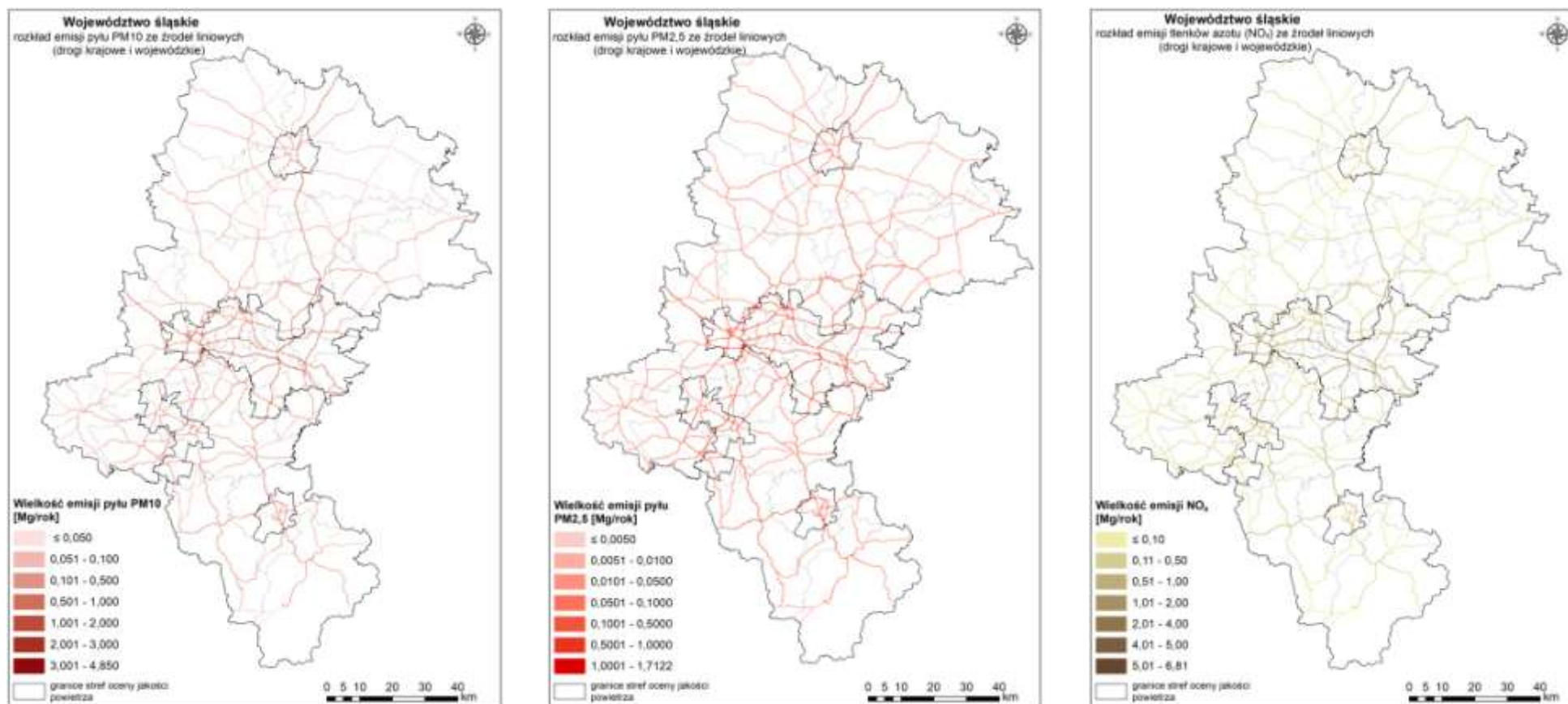
Rysunek 91. Rozkład przestrzenny emisji pyłu PM10, PM2,5 oraz tlenków azotu z dróg krajowych i wojewódzkich w województwie śląskim w roku bazowym 2015
