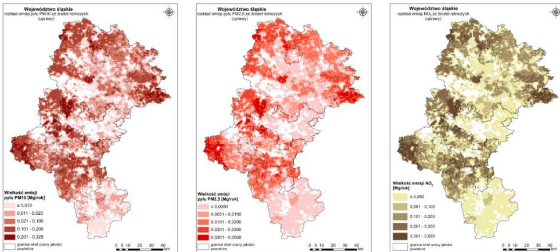
Rysunek 97. Rozkład przestrzenny emisji pyłu zawieszonego PM10 i PM2,5 oraz tlenków azotu z obszarów upraw w siatce obliczeniowej na terenie województwa śląskiego w roku bazowym 2015
