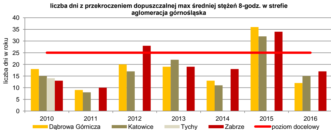
Rysunek 13. Liczba dni z przekroczeniem dopuszczalnej maksymalnej 8-godzinnej średniej kroczącej dla ozonu w punktach pomiarowych w strefie aglomeracja górnośląska w latach 2010-2016 74
