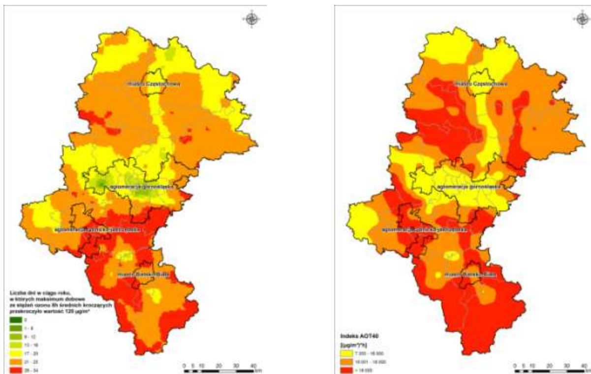
Rysunek 56. Rozkład przestrzenny wartości kryterialnych dla ozonu ze względu na ochronę ludzi oraz ochronę roślin na terenie województwa śląskiego w roku bazowym 2015
