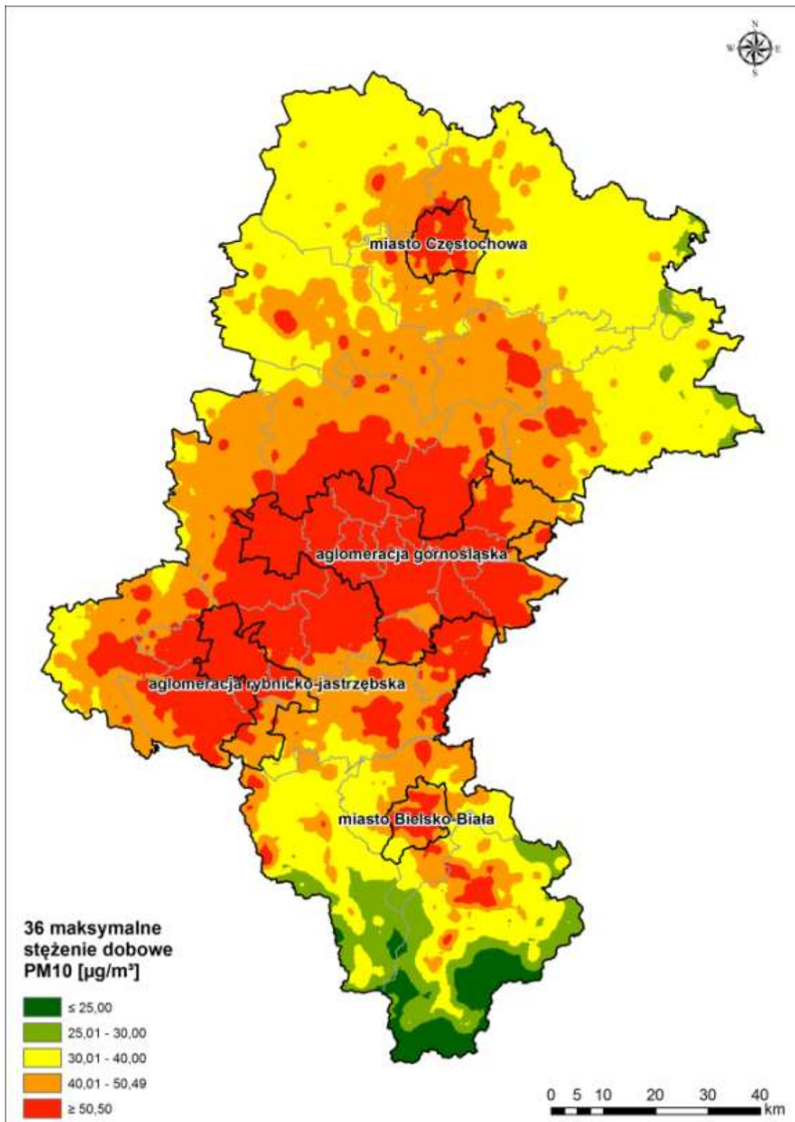
Rysunek 171. Rozkład 36-tego maksymalnego stężenia 24-godzinne pyłu PM10 w województwie śląskim w roku bazowym 2015
