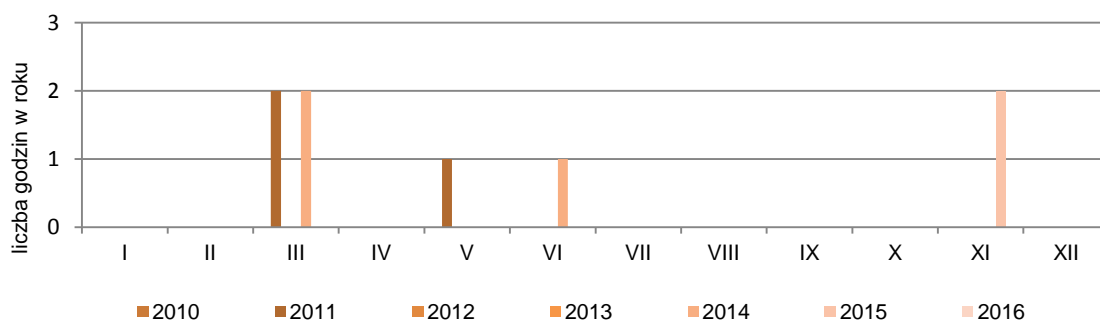
liczba godzin z przekroczeniem dopuszczalnej wartości godzinowej NO 2 w Katowicach
