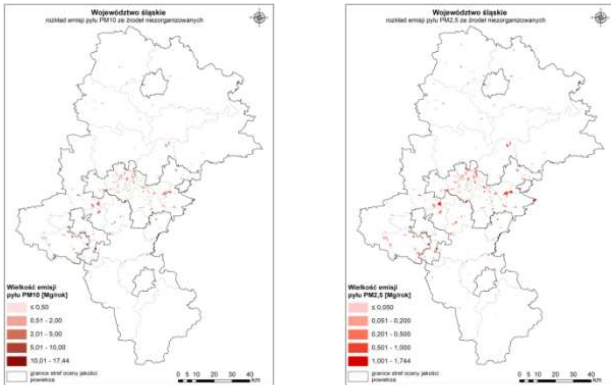
Rysunek 94. Rozkład przestrzenny wielkości emisji pyłu zawieszonego PM10 i PM2,5 ze źródeł niezorganizowanych w siatce obliczeniowej na terenie województwa śląskiego w roku bazowym 2015
