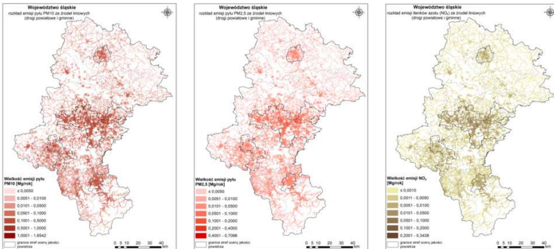
Rysunek 92. Rozkład przestrzenny emisji pyłu PM10, PM2,5 oraz tlenków azotu z dróg powiatowych i gminnych w siatce obliczeniowej w województwie śląskim w roku bazowym 2015
