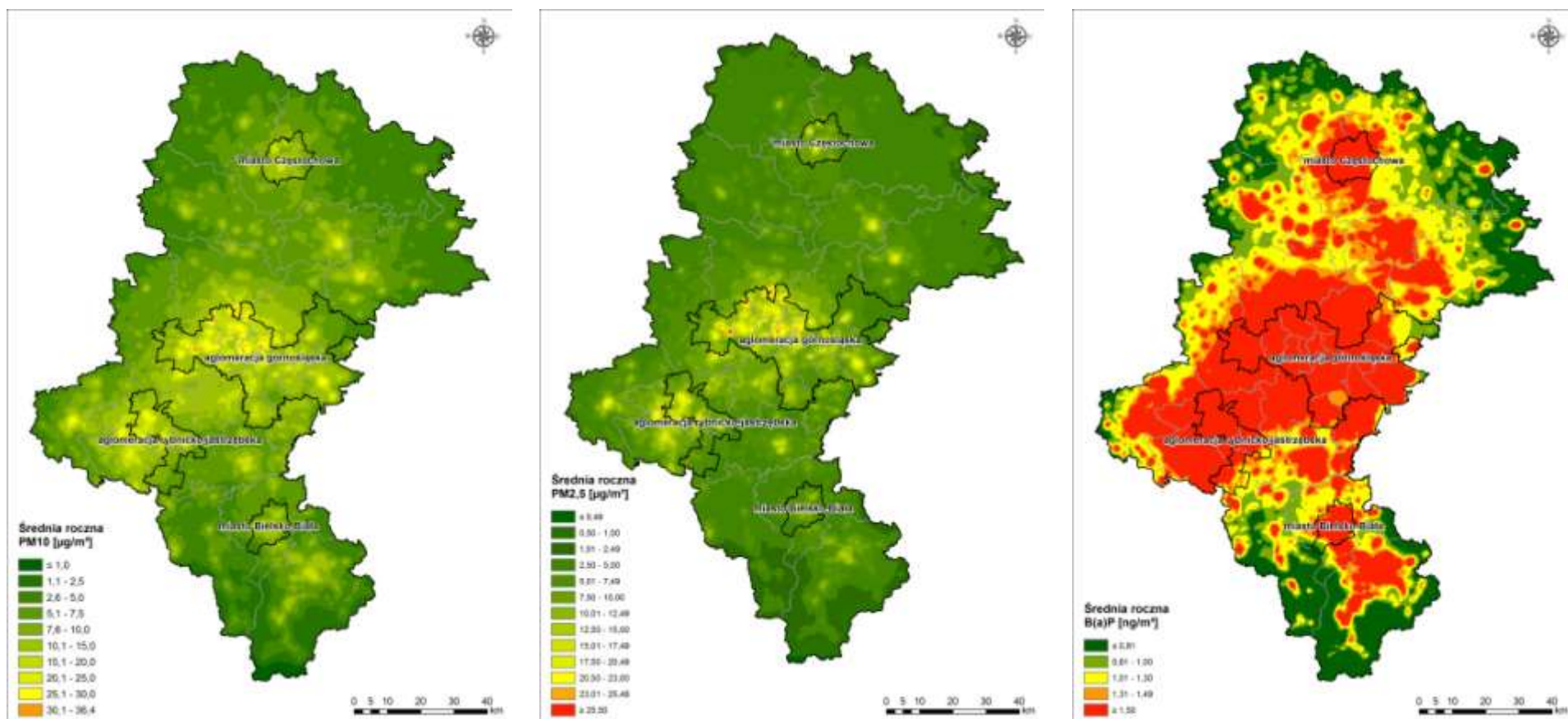
Rysunek 62. Rozkład stężeń średniorocznych pyłu PM10, PM2,5 oraz B(a)P generowanych przez źródła powierzchniowe w województwie śląskim 152
