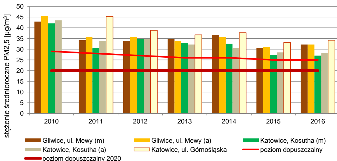
stężenie średnioroczne PM 2,5 w strefie aglomeracja górnośląska
