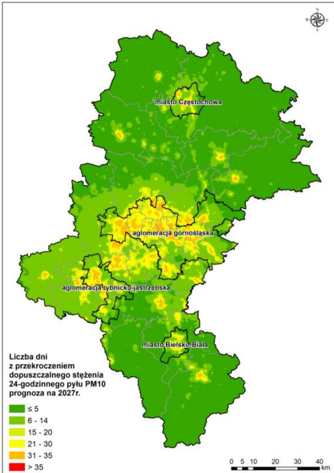
Rysunek 179. Rozkład liczby dni z przekroczeniem dopuszczalnego poziomu 24-godzinne dla pyłu PM10 w województwie śląskim w roku prognozy 2027
