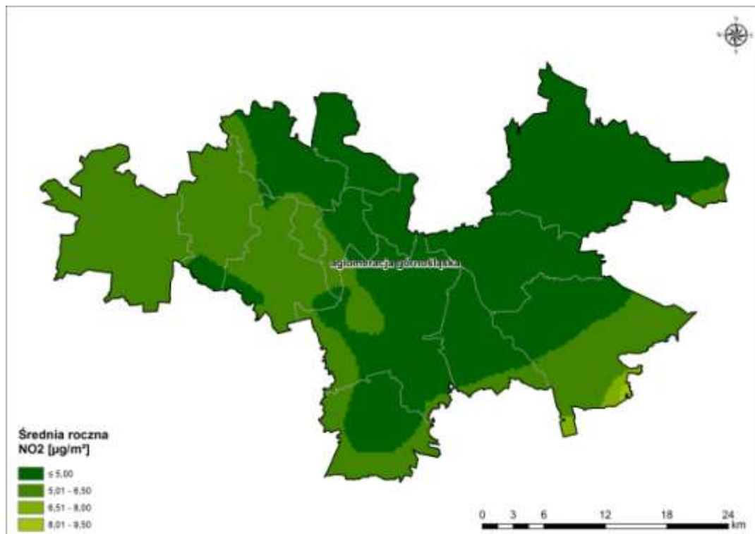
Rysunek 71. Rozkład stężeń średniorocznych \text{NO}_2 tło ponadregionalne w aglomeracji górnośląskiej 161
